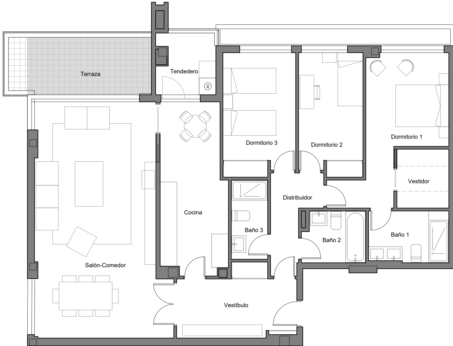
ESQUEMA LOCALIZACIÓN PLANTA 1ª
